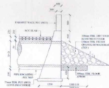
DETAIL-A (SCALE 1:50)
